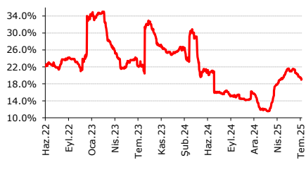
DOAS
