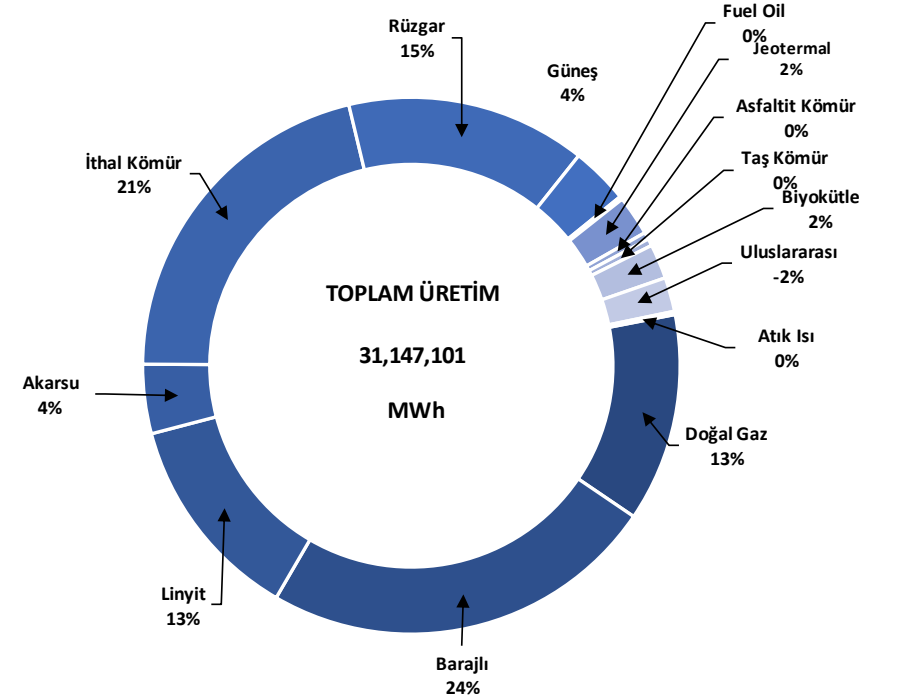
Toplam üretilen elektriğin kaynaklara göre dağılımı | Ağustos 2026
