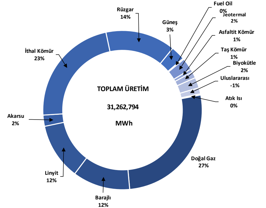
Toplam üretilen elektriğin kaynaklara göre dağılımı | Ağustos 2025
