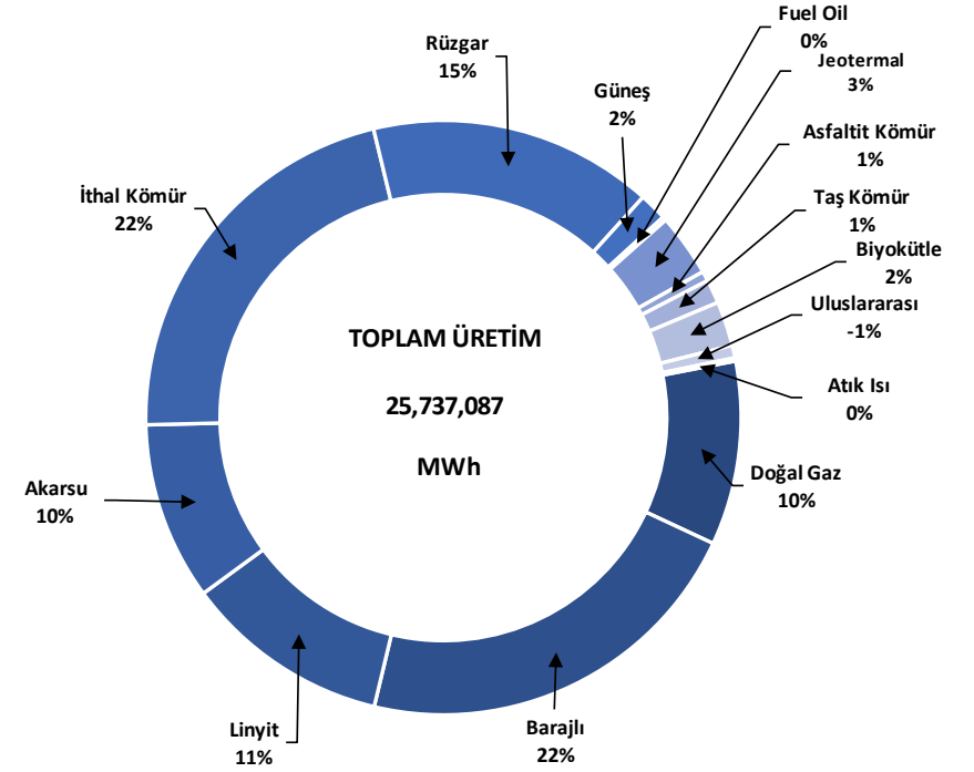
Toplam üretilen elektriğin kaynaklara göre dağılımı | Şubat 2026
