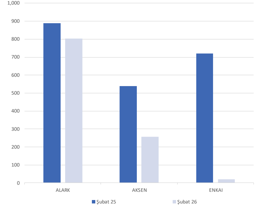
Karşılaştırmalı toplam elektrik üretimi (GWh) | Şubat
