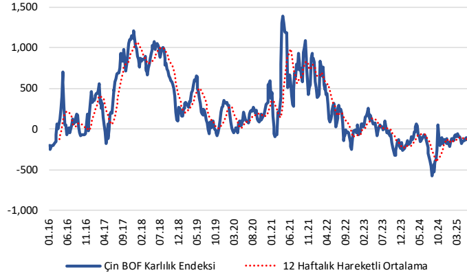
Çin Bazık Oksijen Fırın Çelik Üreticileri Karlılık Endeksi (CNY/ton)
