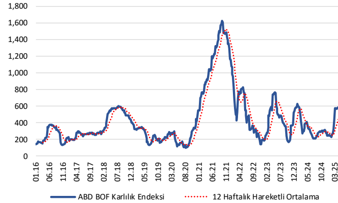
ABD Bazık Oksijen Fırın Çelik Üreticileri Karlılık Endeksi (USD/ton)
