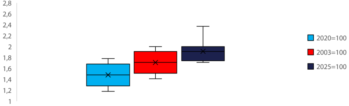
Grafik-1: PUSULA TÜFE ARIMA (Açık mavi 2020, kırmızı 2003, lacivert 2025'e endeksli, %)
