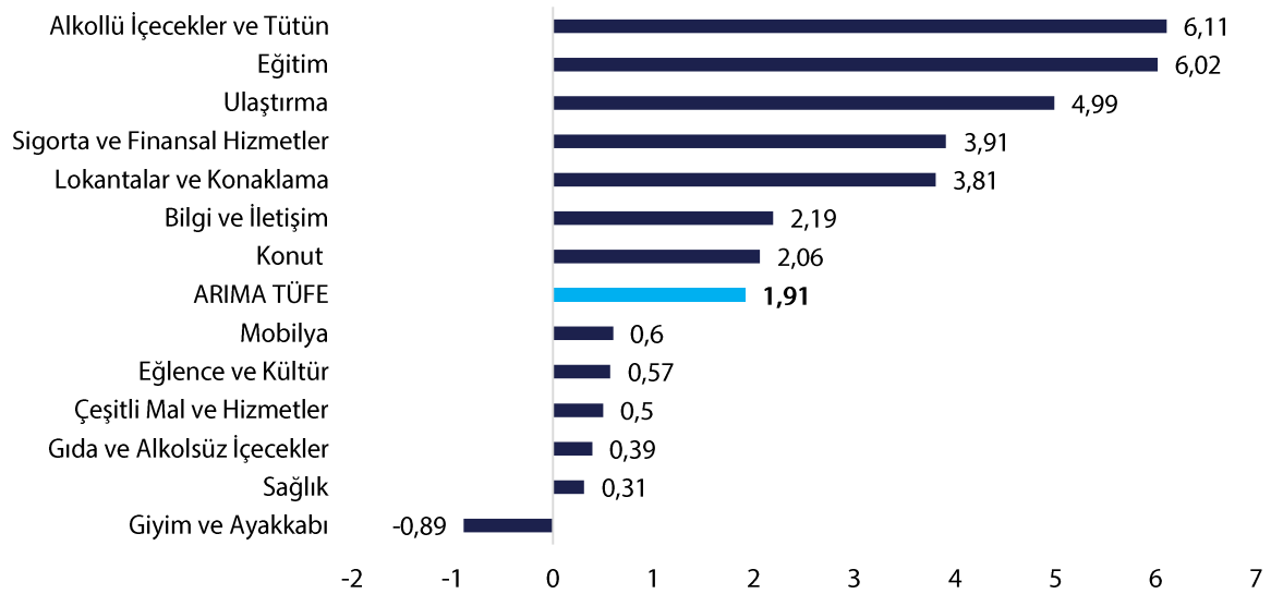
Grafik-2: Gruplar bazında ARIMA (seviye, %, %1,91 üzerinden)
