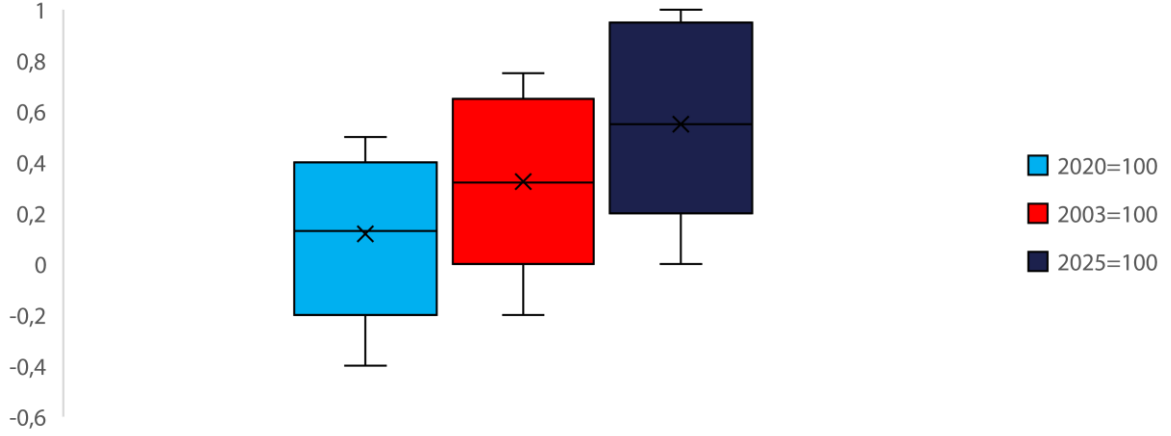
Grafik-2: Gruplar bazında ARIMA (seviye, %, % üzerinden)
