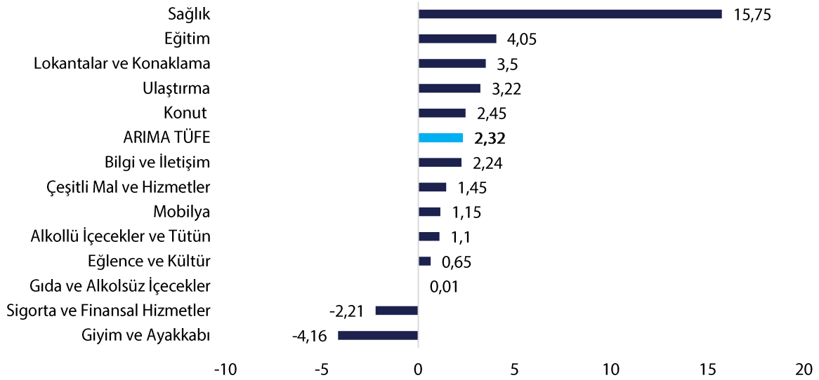
Grafik-2: Gruplar bazında ARIMA (seviye, %, %2,32 üzerinden)
