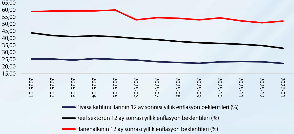
Grafik-1: Sektörel TÜFE Beklentileri (% seviye)
