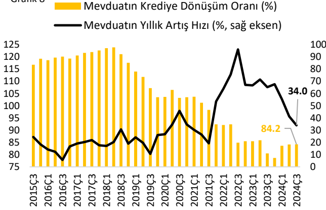
Grafik 8
