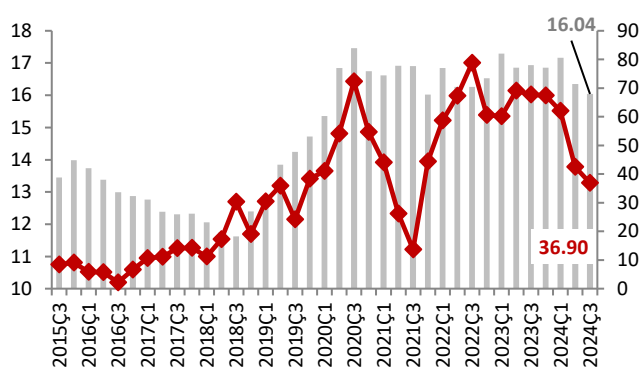
Grafik 6 MDP/Aktifler
