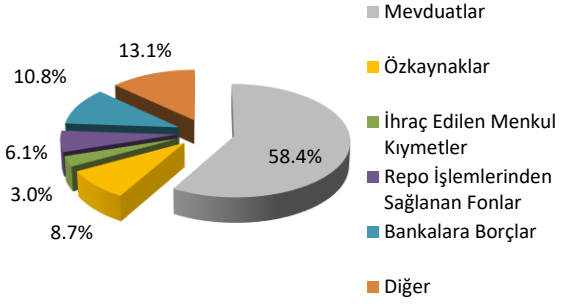
Grafik 7
