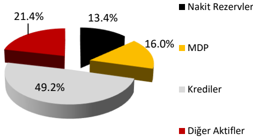
Toplam Aktifler
